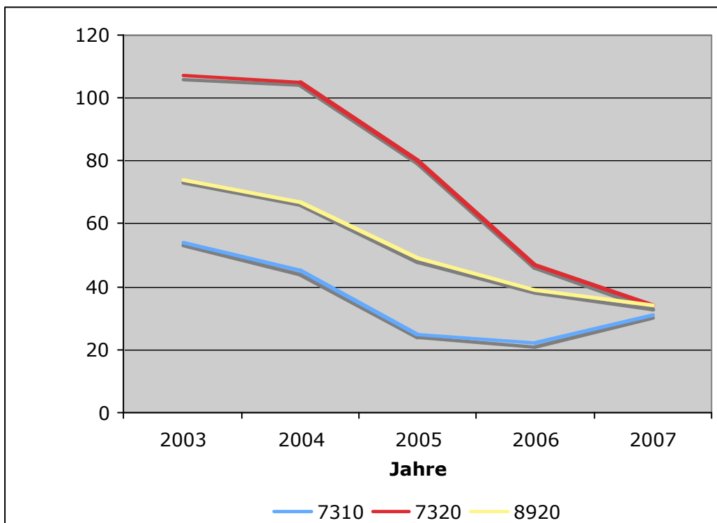
Abbildung 13: Zeitreihen III: 7310, 7320, 8920
