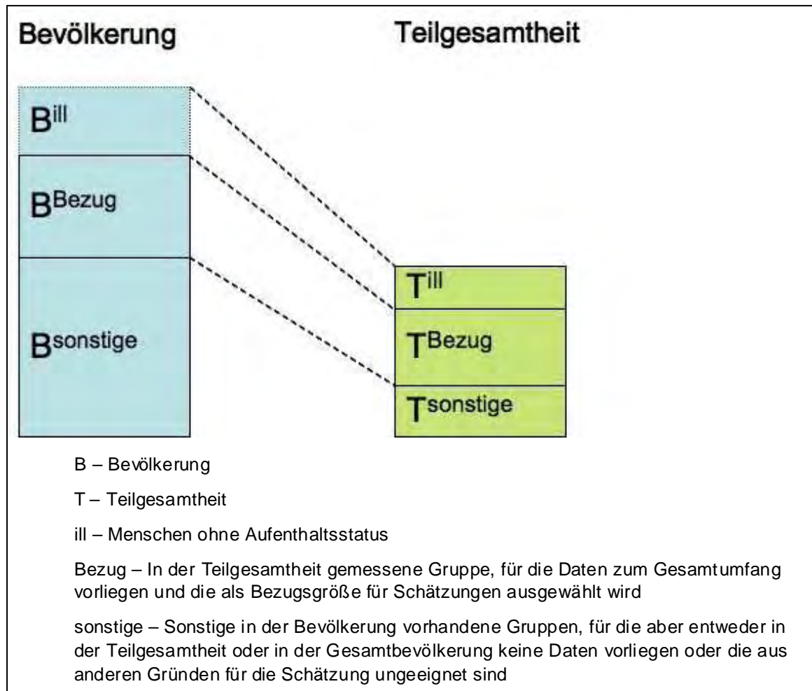
Abbildung 1: Multiplikatorlogik
